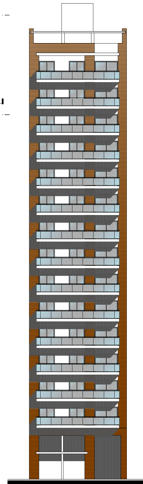
VISTA FRENTE
