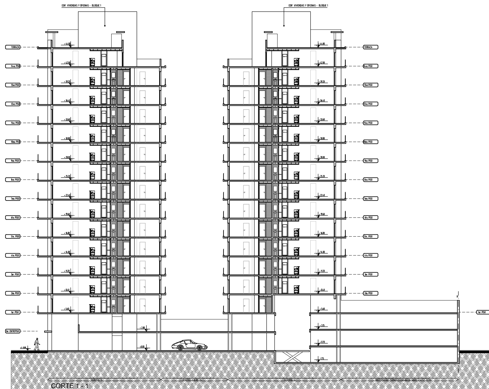
CORTE LONGITUDINAL 1 - 1
